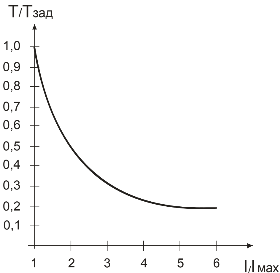
Рисунок 9 – временная характеристика защитного отключения реле по току перегрузки
