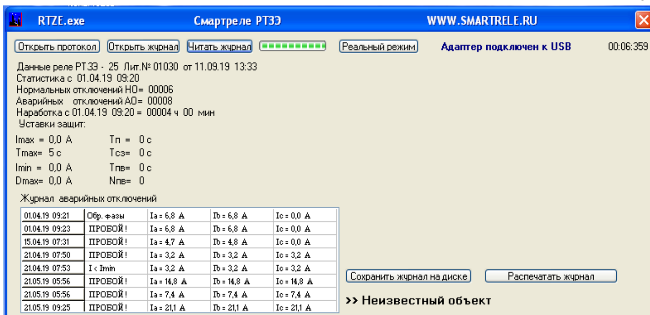
Рисунок 8 - отображение журнала событий Смартреле РТЗЭ на экране ПК
